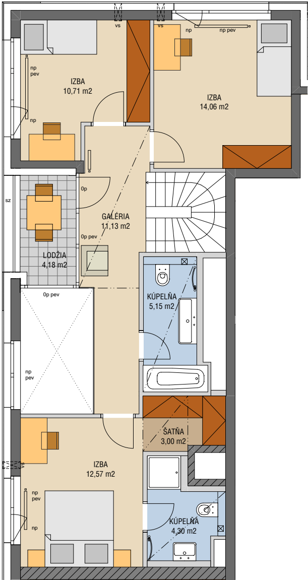
HORNÉ PODLAŽIE
