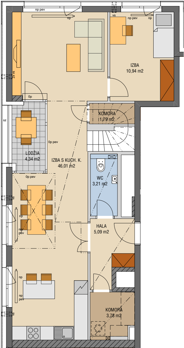
DOLNÉ PODLAŽIE
