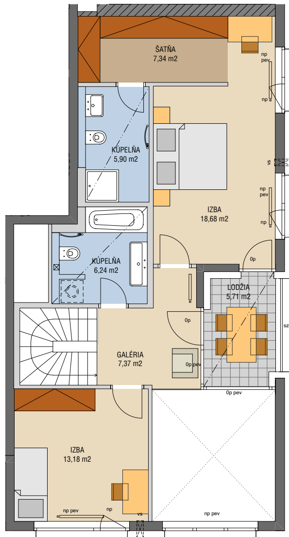
HORNÉ PODLAŽIE
