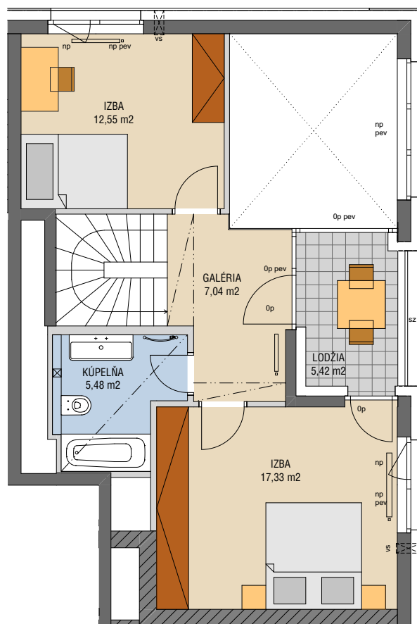
HORNÉ PODLAŽIE
