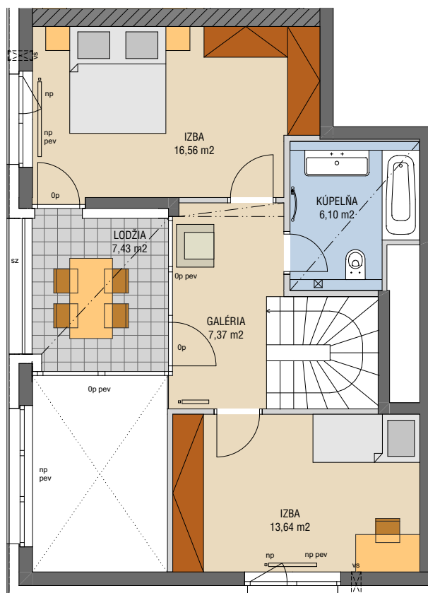
HORNÉ PODLAŽIE
